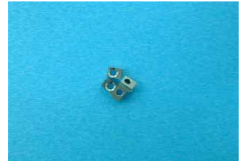
レンズホルダー 材質 SUS304
